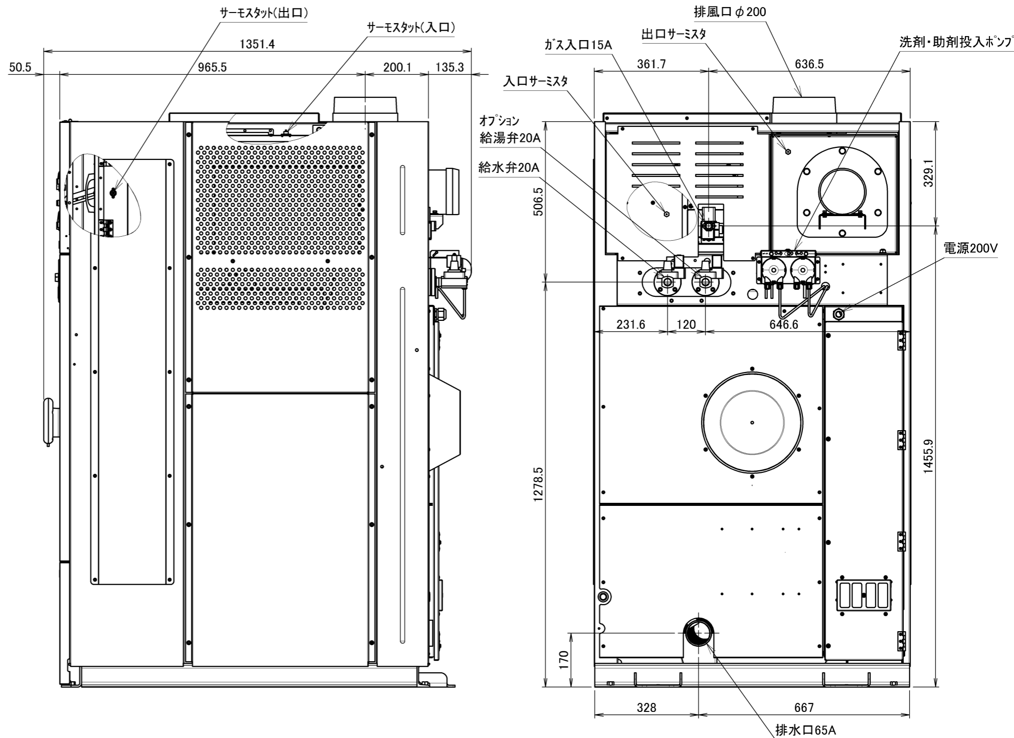
コイン洗濯乾燥機 WD272CS 外観図
