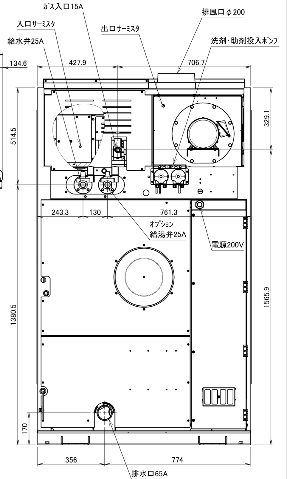
コイン洗濯乾燥機 WD352CS 外観図
